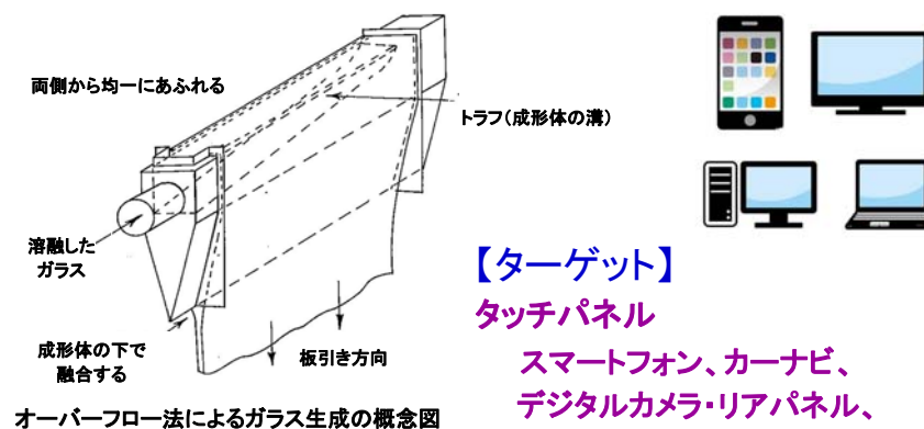
オーバーフロー法によるガラス生成の概念図
