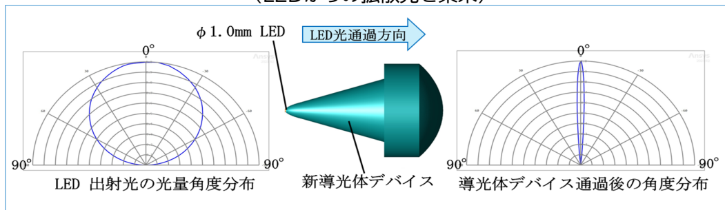
本デバイスの機能例 (LEDからの拡散光を集束)
