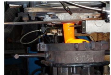
溶融ガラスを金型に供給する様子
