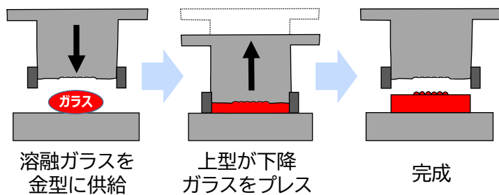
ダイレクトプレス成型のイメージ図
