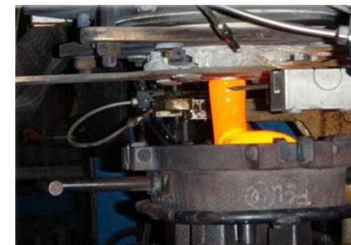
溶融ガラスを金型に供給する様子
