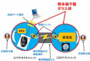
江戸っ子1号の構成図
